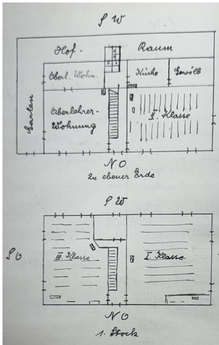
Půdorys školy 1872
